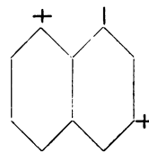
s Disulfosäure. D. R. P. 55 094. Ber. 22. 3382.
